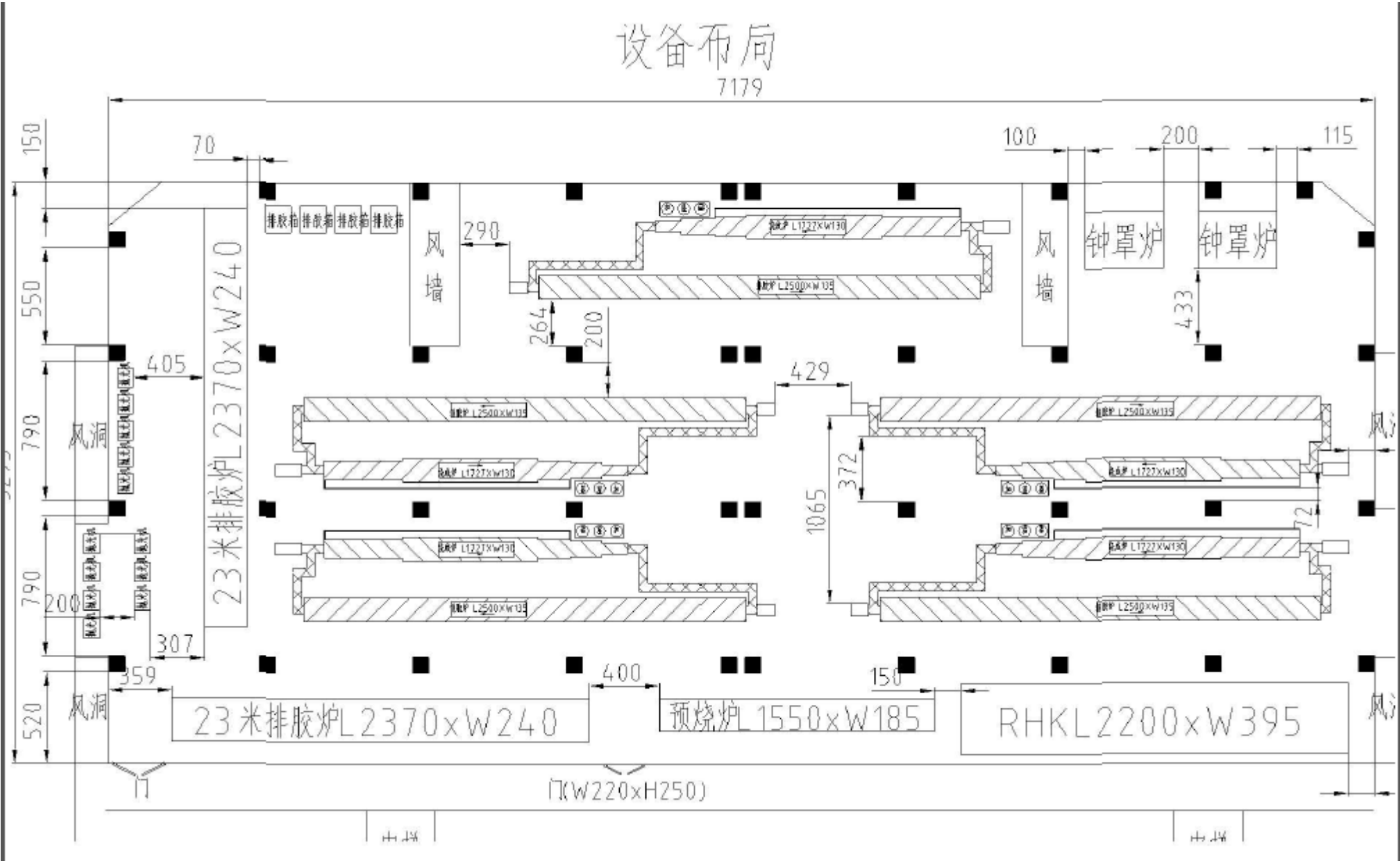
图 6：烧炉车间
