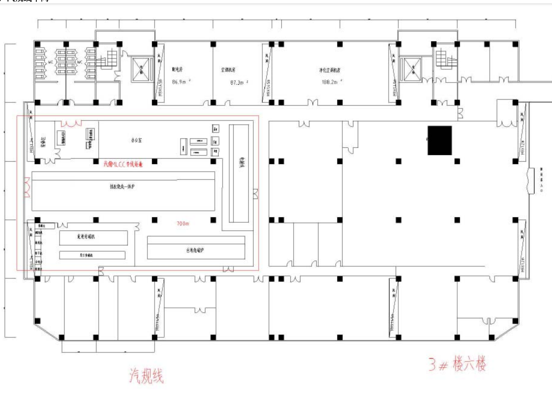
图 3：汽规线车间
