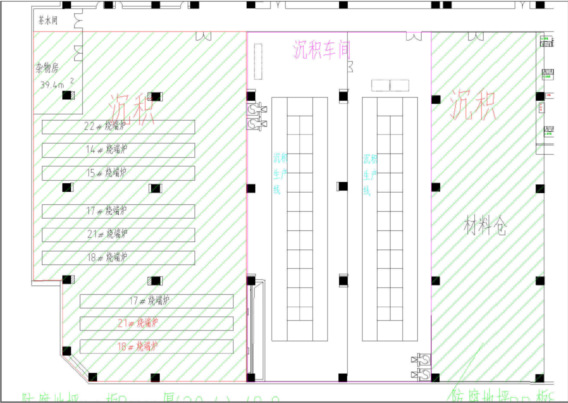
图 10：沉积车间
